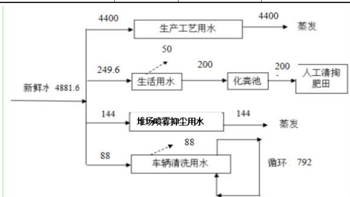
图 1-1 项目水平衡图 (单位: m 3 /a)
