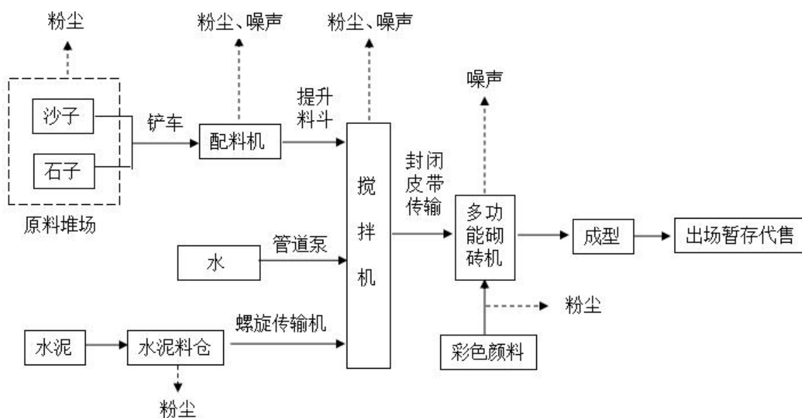
图 5-1 水泥砖、水泥花砖工艺流程及产污环节图
