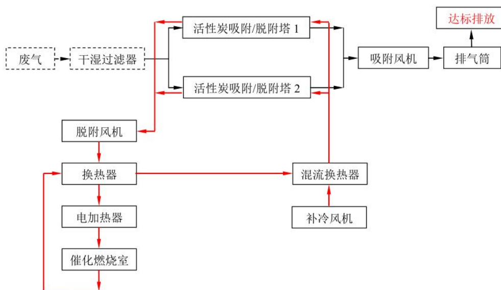
图五 催化燃烧设备工艺流程图
