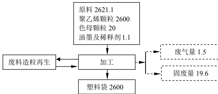
图二 本项目物料平衡图 (单位: t)
