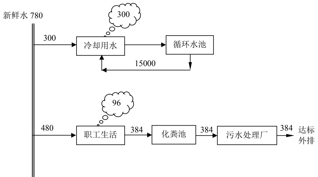
图一 本项目水平衡图 (单位: \text{m}^3/\text{a} ; ☁ 表示蒸发损失量)
