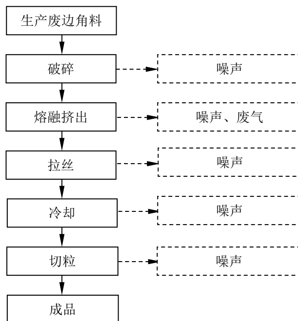
图四 造粒工艺流程图
