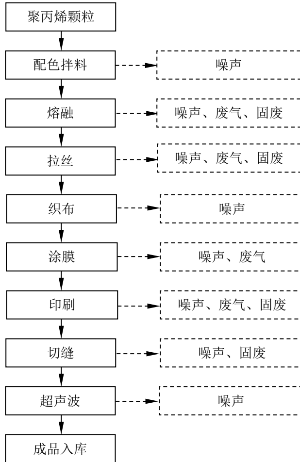
图四 编织袋生产工艺流程图
