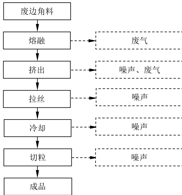
图五 编织袋造粒工艺流程图
