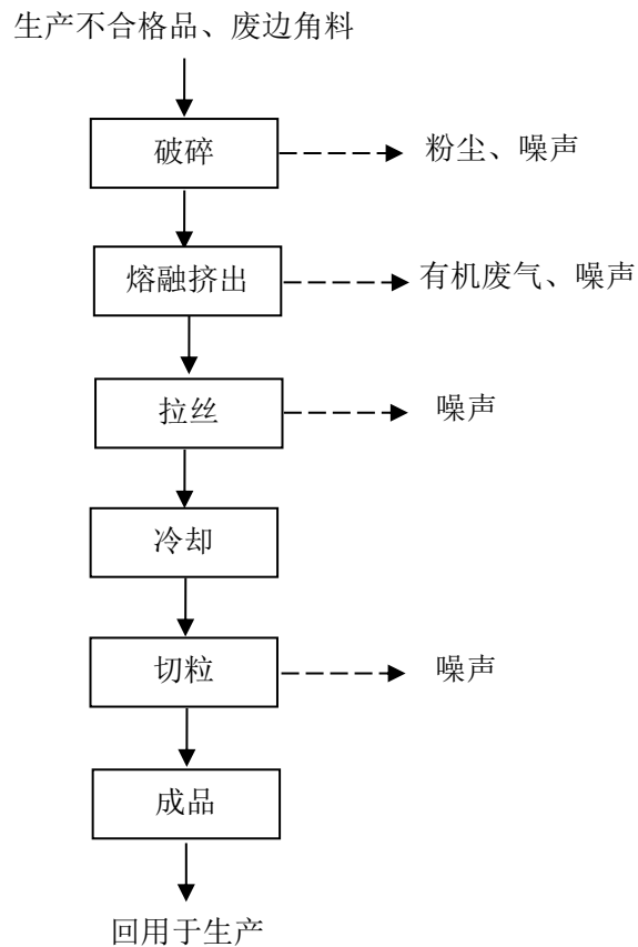
图 2-4 制粒生产工艺流程及产污环节图
