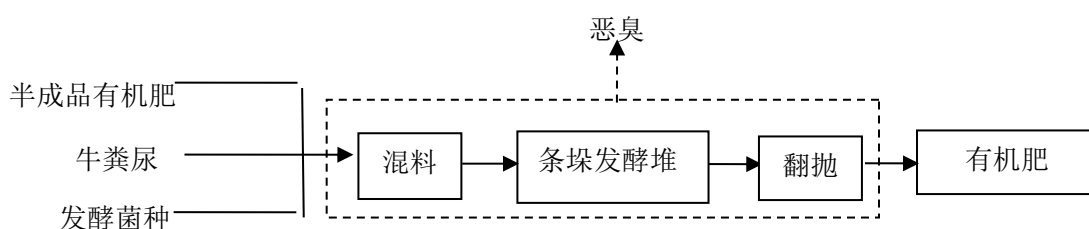
图 2.2-5 制肥工艺流程图
