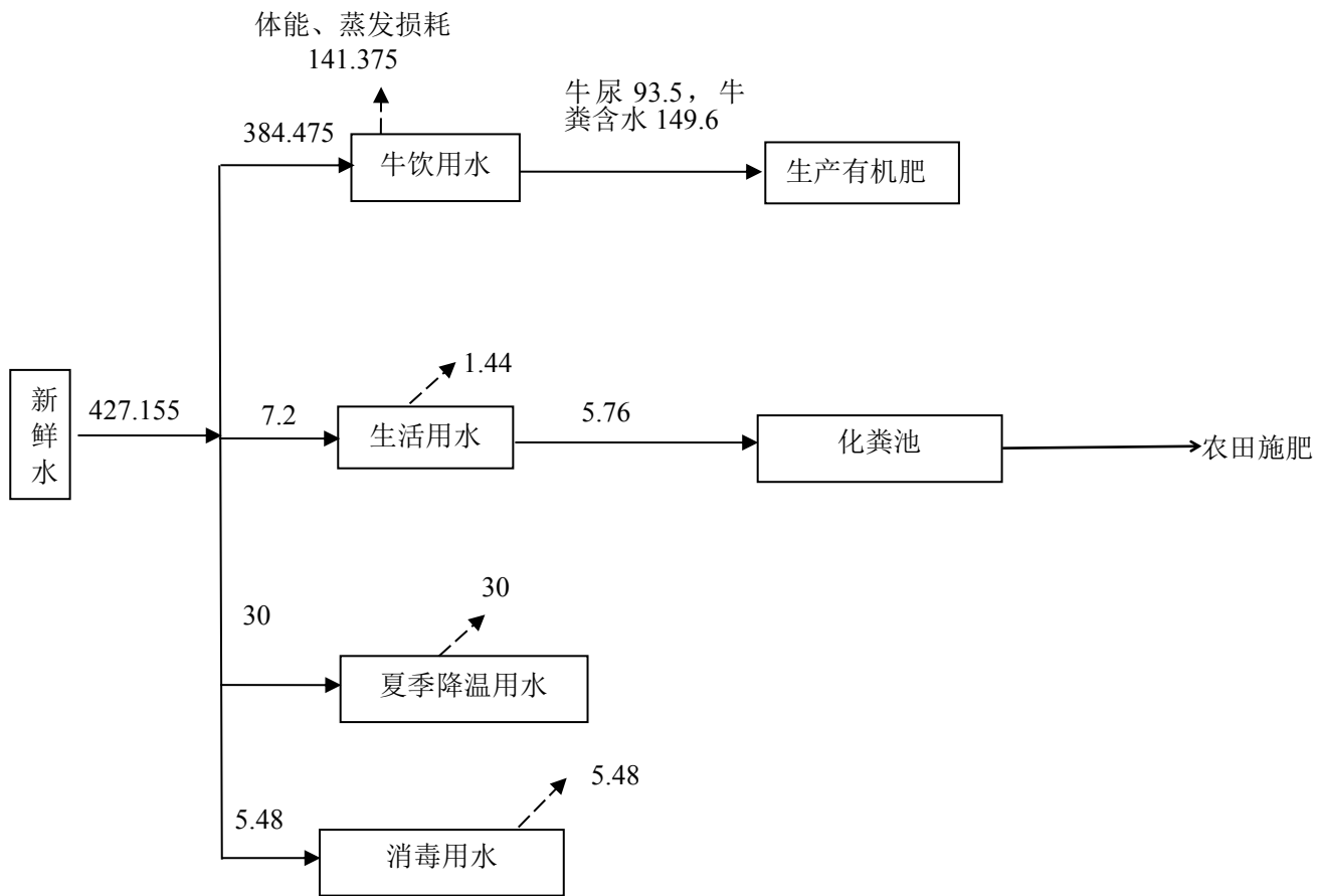
图 2.1-2 本项目夏季水平衡图 (单位: m 3 /d) (122 天)
