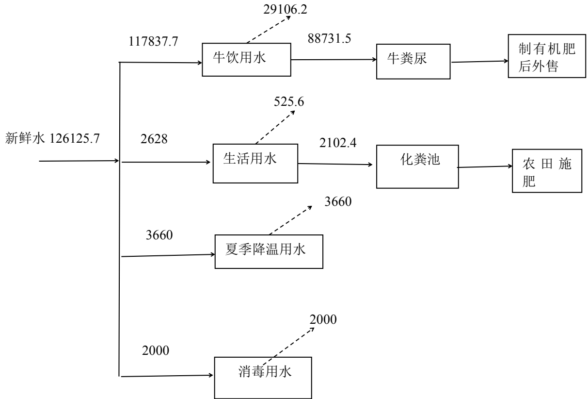
图 2.1-1 项目全年水平衡图 (单位: \text{m}^3/\text{a} )
