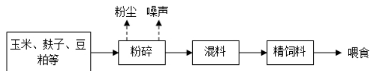
图 2.2-1 精饲料加工工艺流程图
