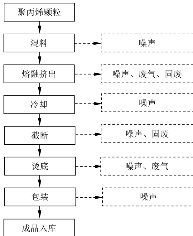
图三 网兜生产工艺流程图
