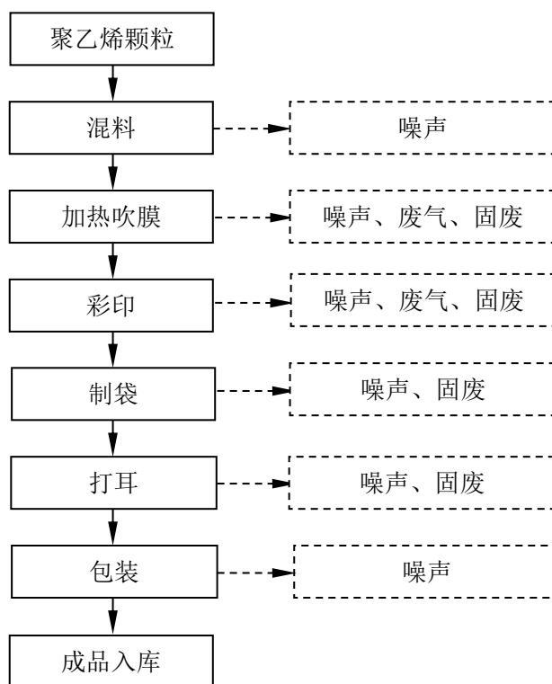
图二 塑料袋生产工艺流程图
