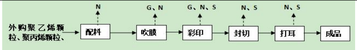
图 2-2 塑料袋生产工艺及产污流程图
