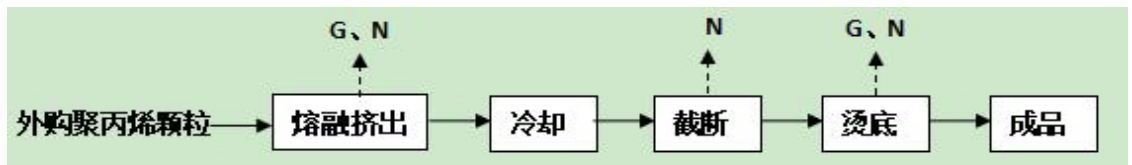
图 2-3 网兜生产工艺及产污流程图
