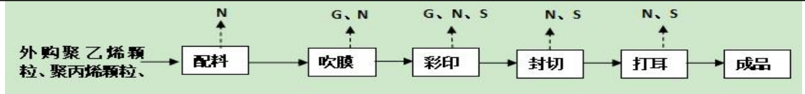
图 2-2 塑料袋生产工艺及产污流程图
