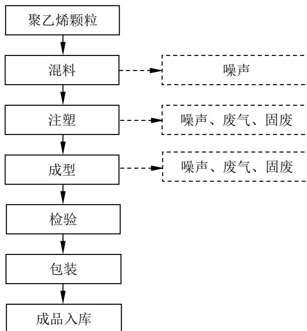
图五 塑料制品生产工艺流程图
