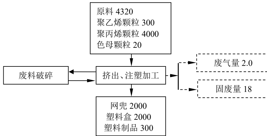
图二 本项目物料平衡图 (单位: t)
