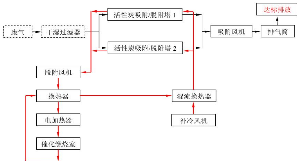
图六 催化燃烧设备工艺流程图
