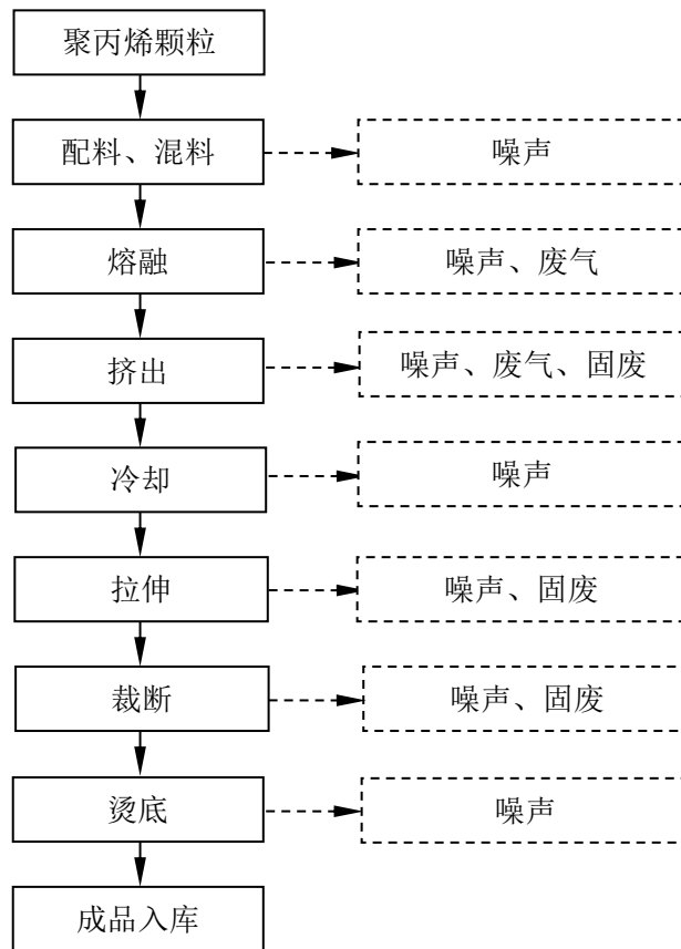
图三 网兜生产工艺流程图
