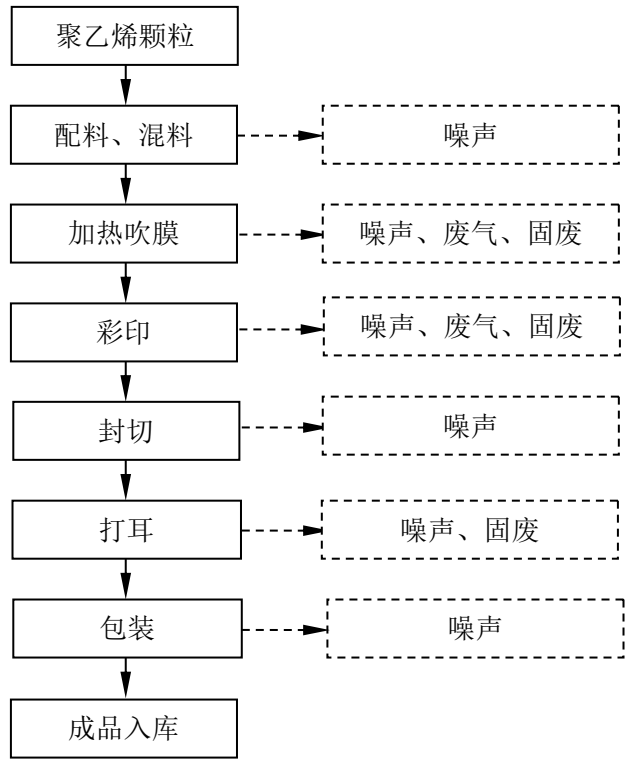
图 2-2 塑料袋制品生产工艺及产污流程图
