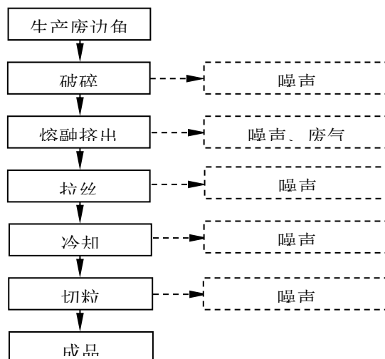
图 2-4 造粒生产工艺及产污流程图
