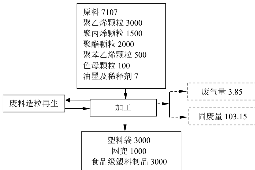
图 2-7 本项目物料平衡图 (单位: t)
