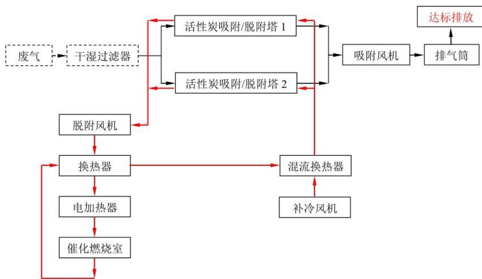
图四 催化燃烧设备工艺流程图
