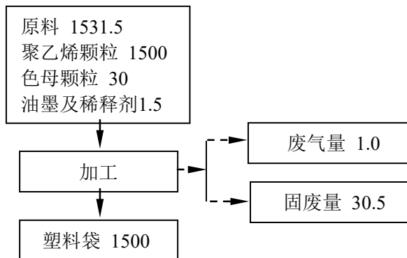
图二 本项目物料平衡图 (单位: t)
