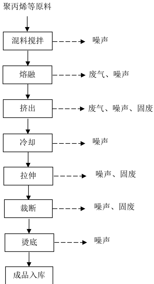
图 2 网兜生产工艺流程及产污环节图
