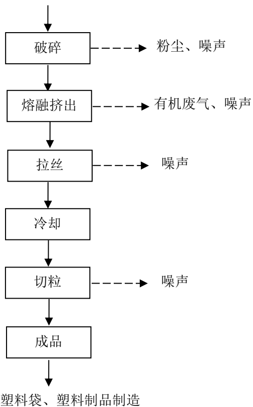
图3 塑料颗粒生产工艺流程及产污环节图
