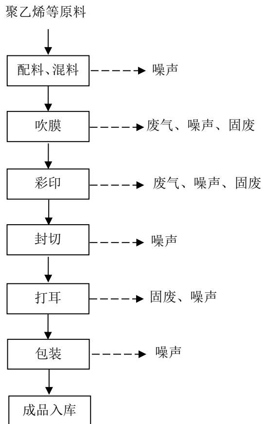
图 2-2 塑料袋生产工艺流程及产污环节图
