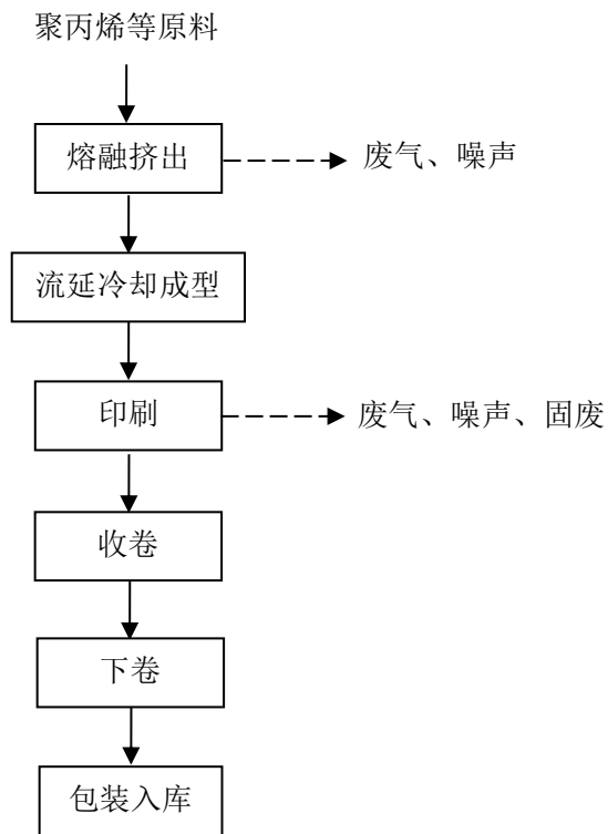
图 2-3 流延膜生产工艺流程及产污环节图
